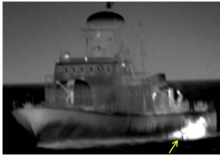
شکل ۱۲. آگزوز و خروجی آب در نمای مایل هدف در تصویر IR در شب با فاصله‌ی تقریبی ۳۵۰ متر
